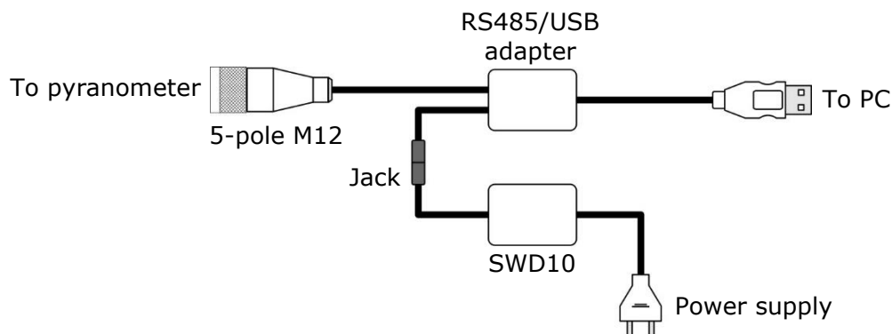
Fig. 4.5: CP24K-5 kit
