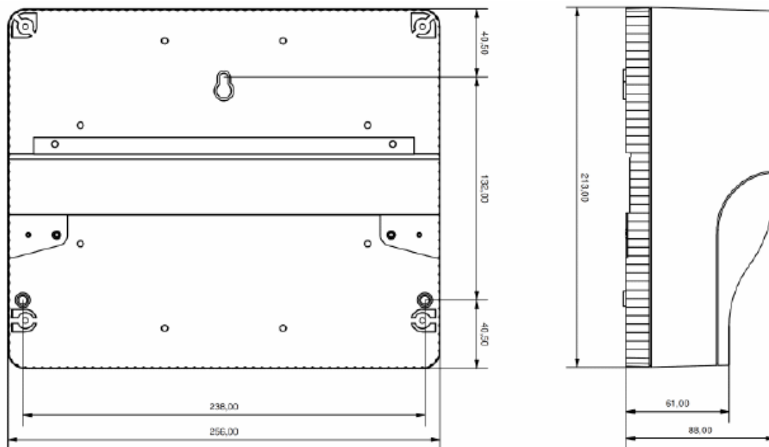
Fig. 1 Dimensions
